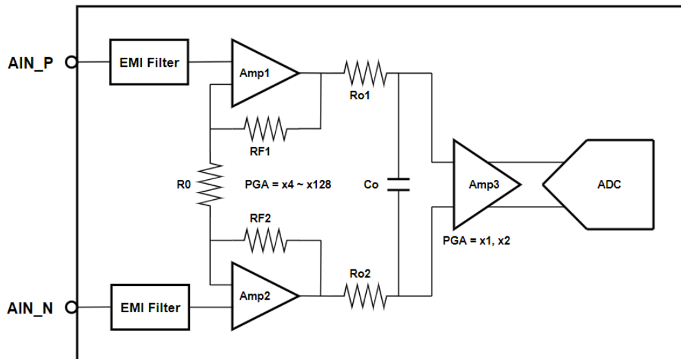
图 3：可编程增益放大器示意图。
