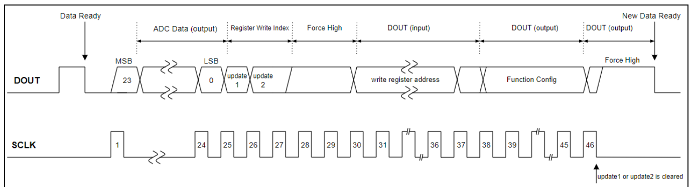
图 11: PMD040 配置时序图（读取程序）
