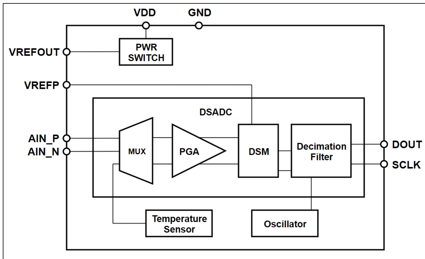
图 1: PMD040 框图
