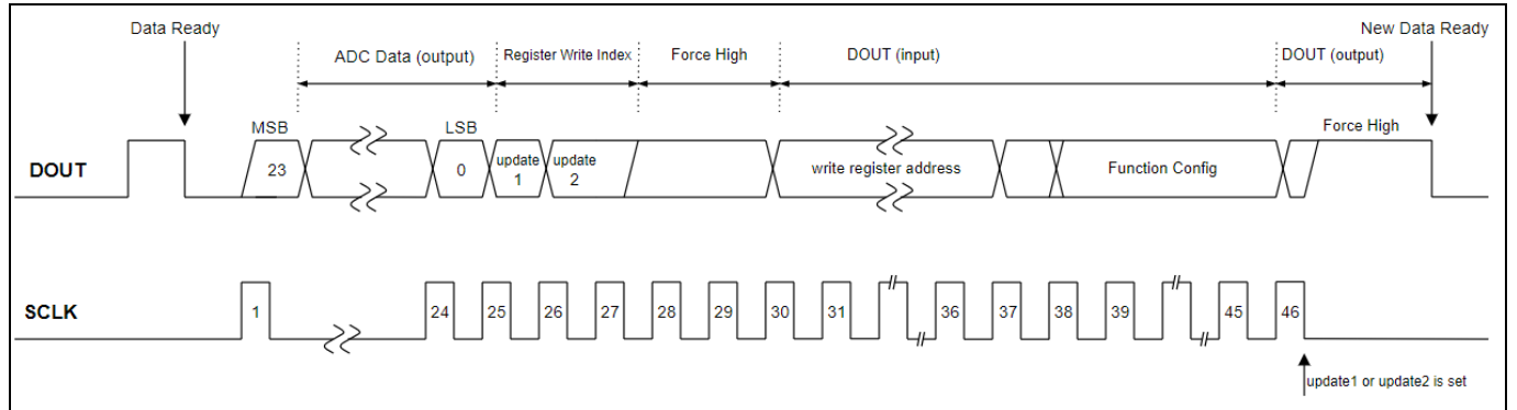
图 10: PMD040 配置时序图（写入程序）
